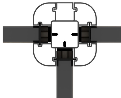
3. T-Kreuz
