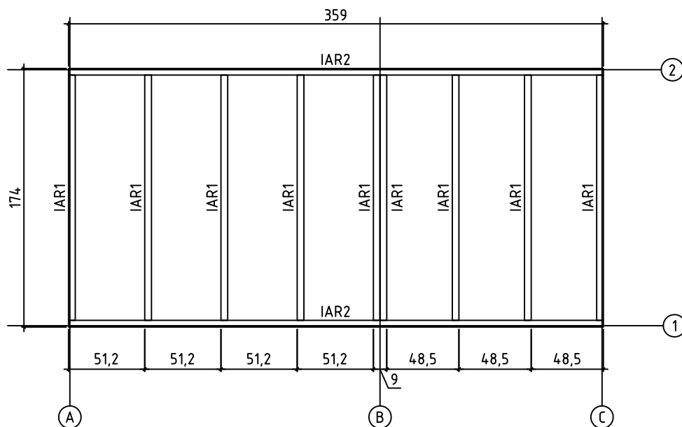
FOUNDATION - FUNDAMENT - FONDATION
