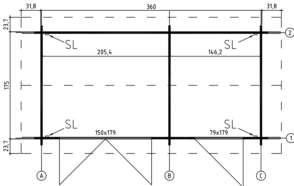
GROUNDPLAN - GRUNDPLAN - PLAN DE MASSE
